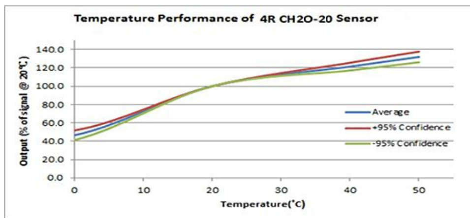
传感器温湿度特性曲线
