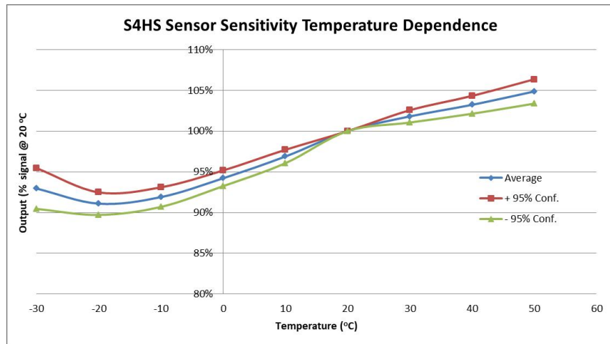
传感器温湿度特性曲线
