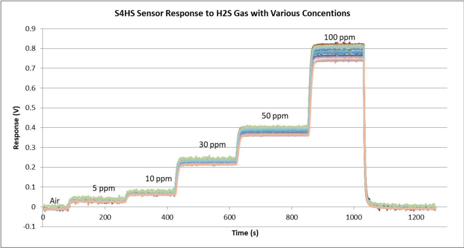
传感器典型的灵敏度特性曲线
