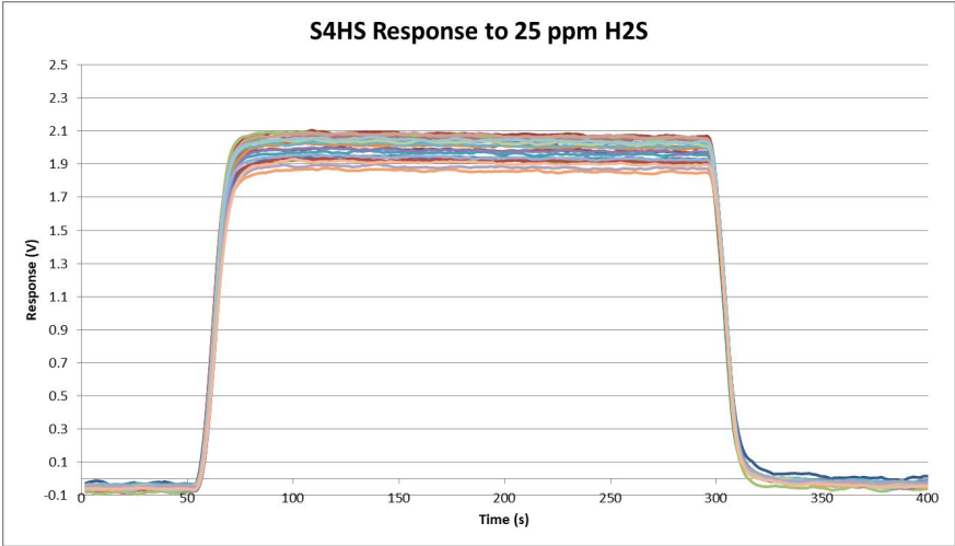
传感器响应恢复曲线
