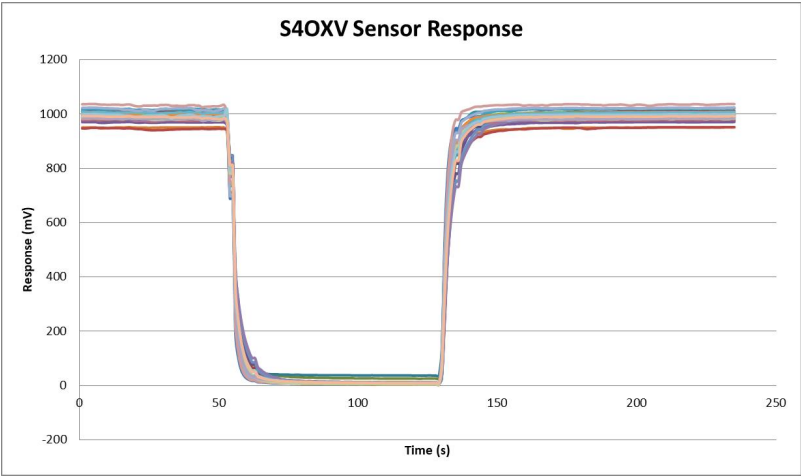
传感器响应恢复曲线
