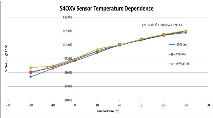
传感器温湿度特性曲线
