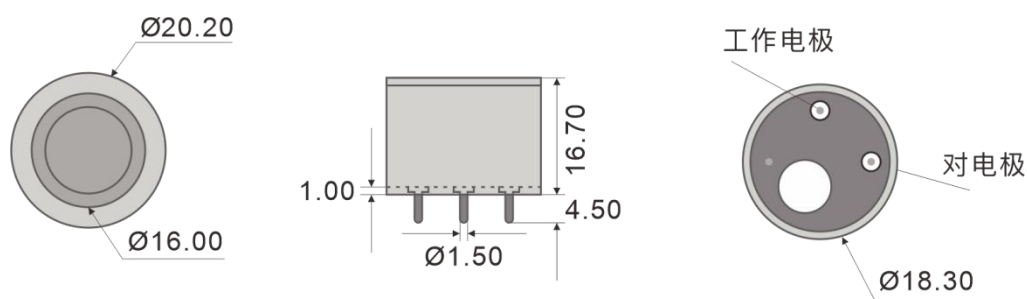
传感器尺寸图
