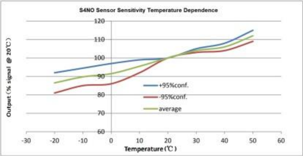
传感器温湿度特性曲线
