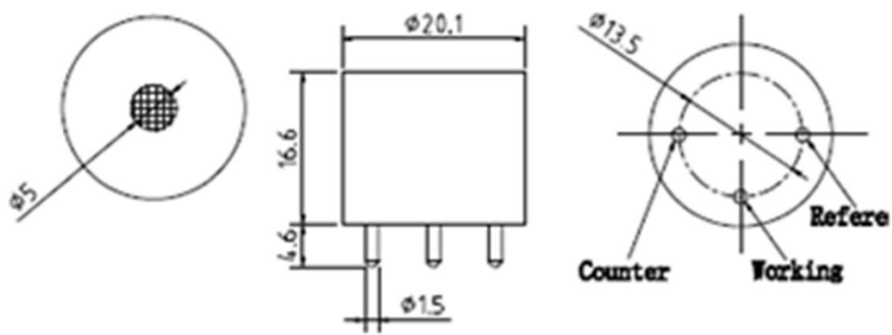
传感器尺寸图
