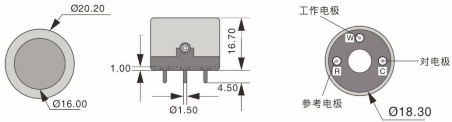
传感器尺寸图
