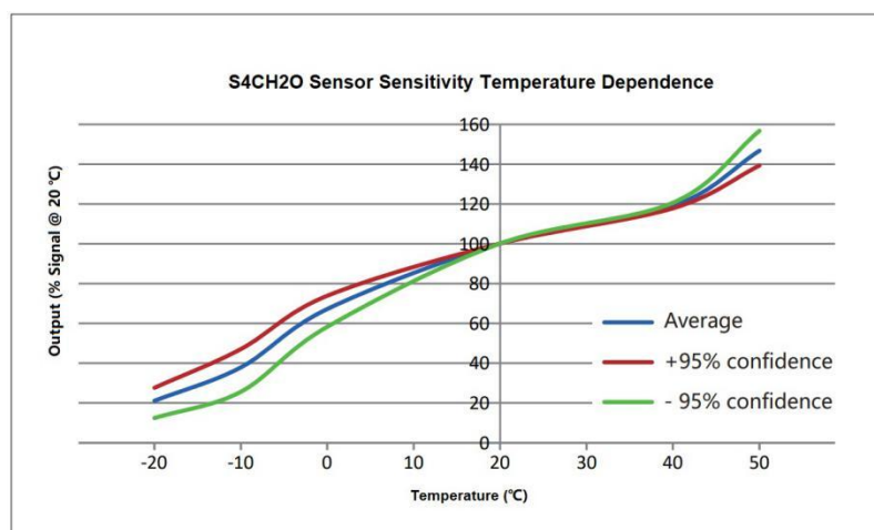
传感器温湿度特性曲线
