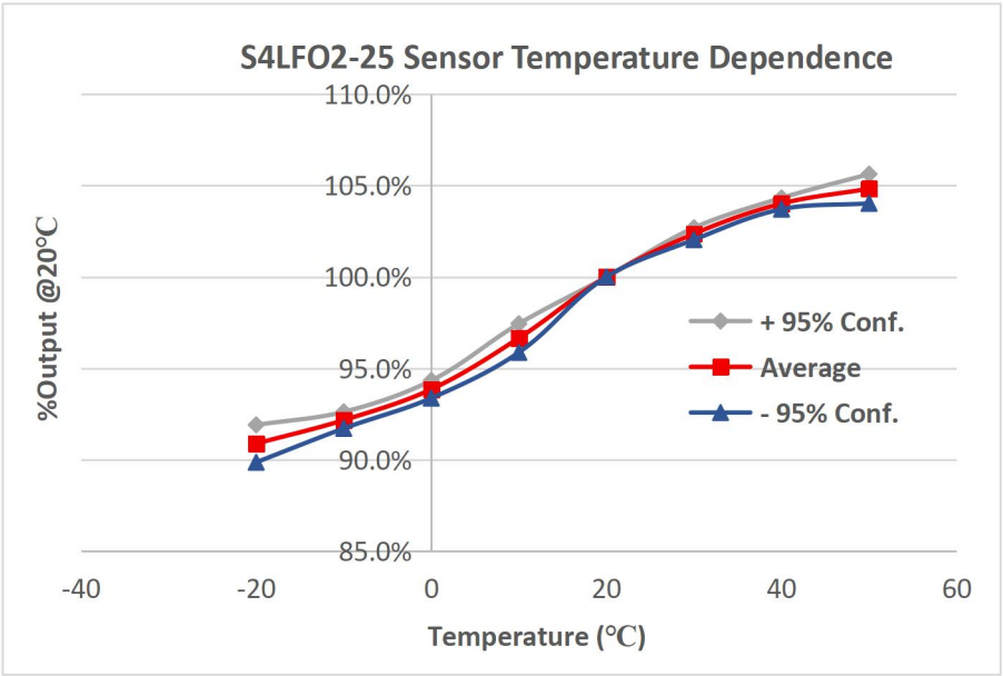
传感器温湿度特性曲线
