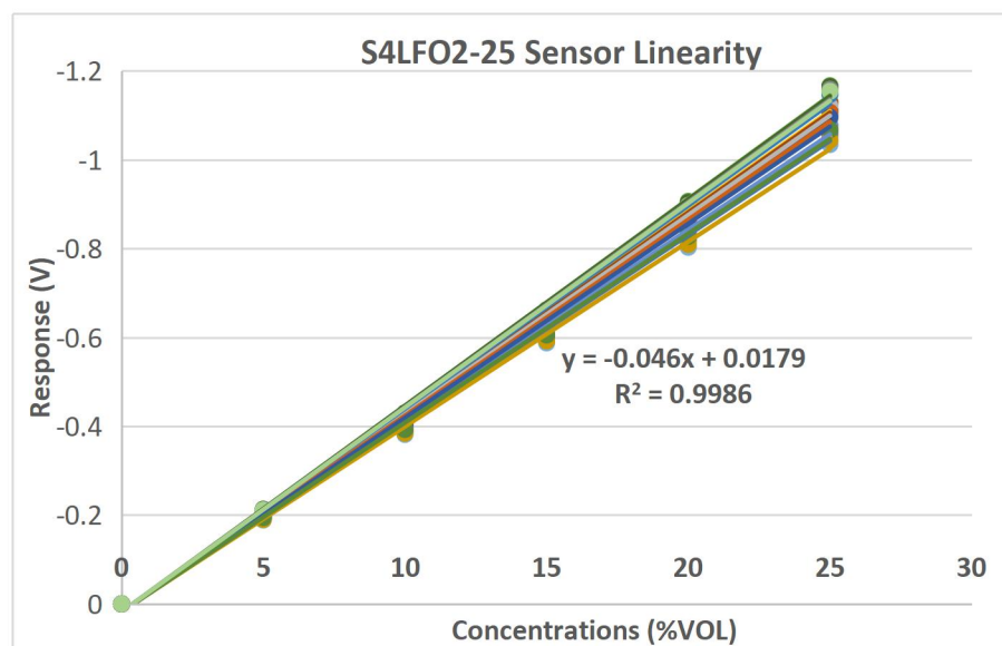
传感器线性拟合曲线
