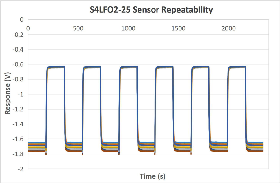
传感器重复性测试曲线
