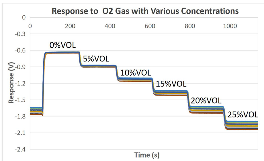
传感器线性测试曲线
