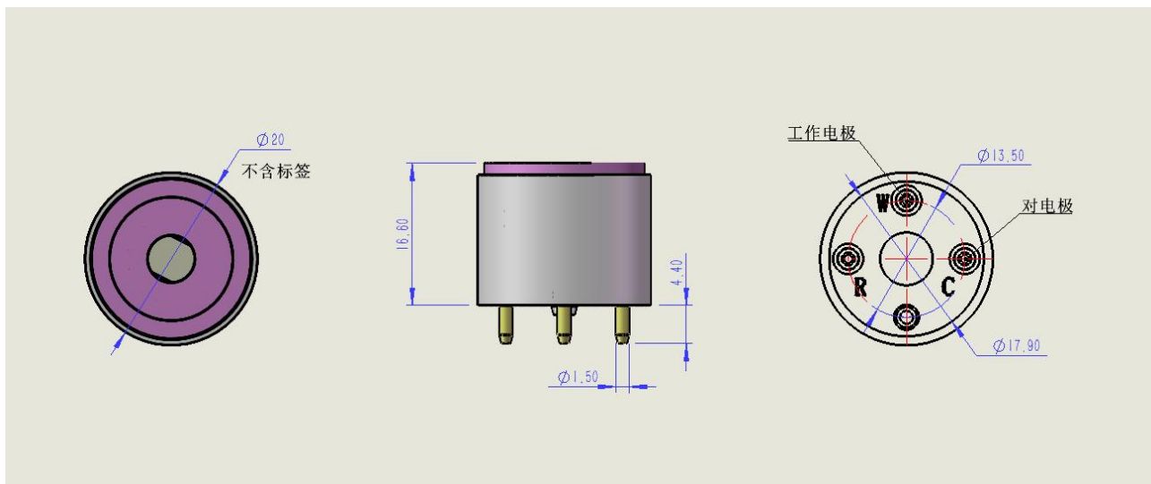
传感器尺寸图
