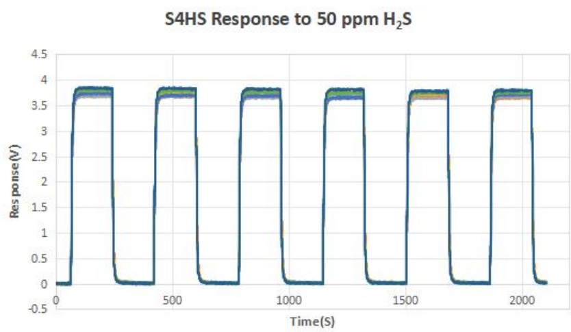
传感器响应重复性曲线
