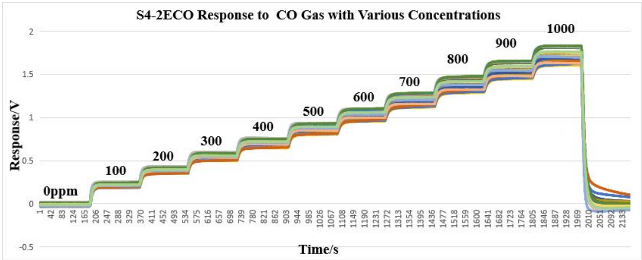
传感器线性响应曲线 (放大电阻 47K)
