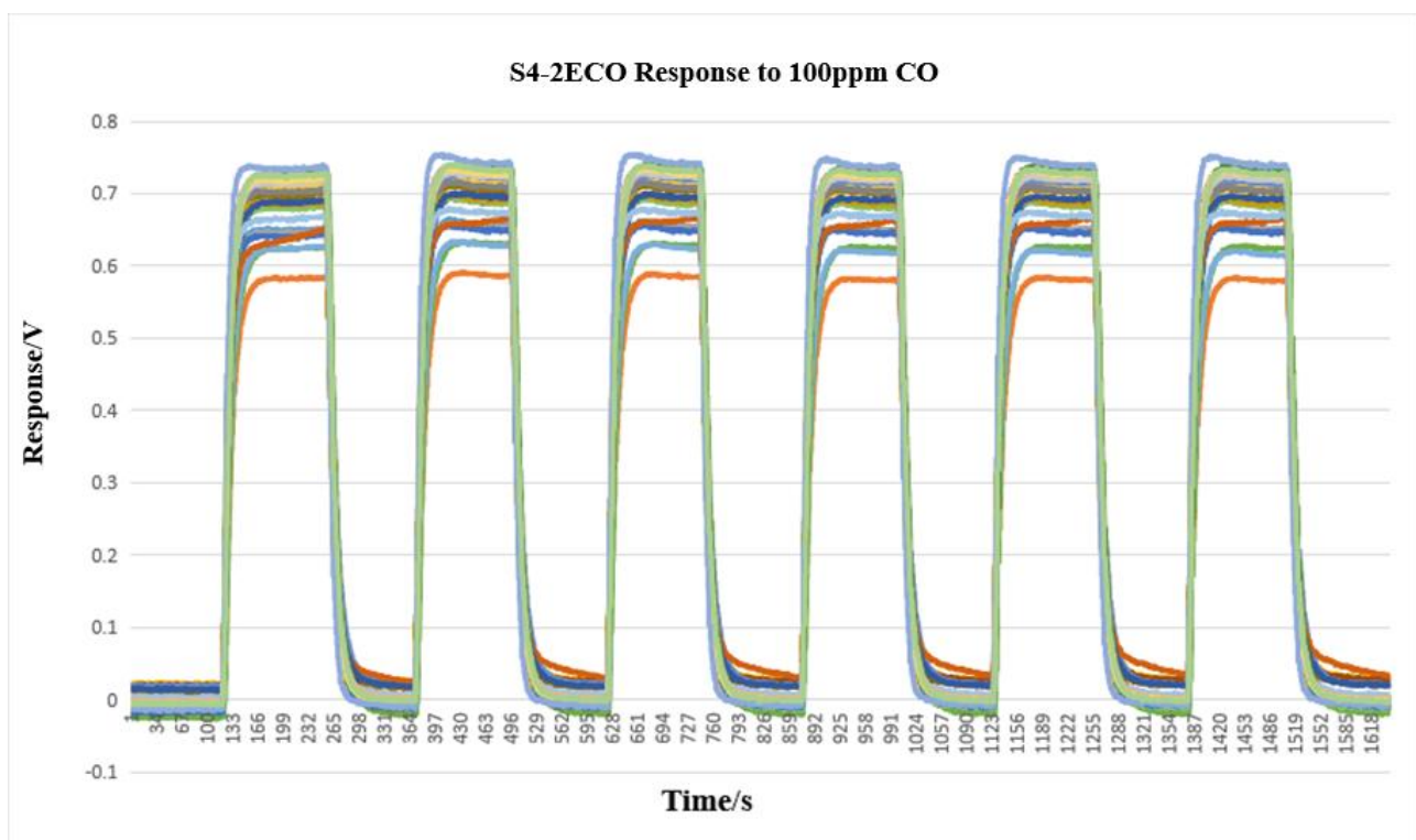
传感器重复性曲线 (放大电阻 150K)
