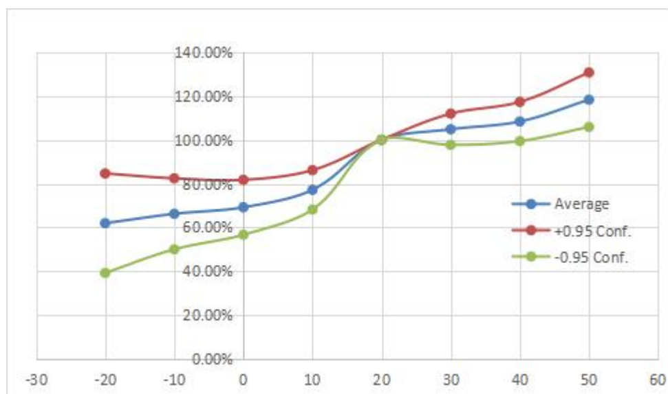
传感器响应温度特性曲线 (放大电阻 150K)
