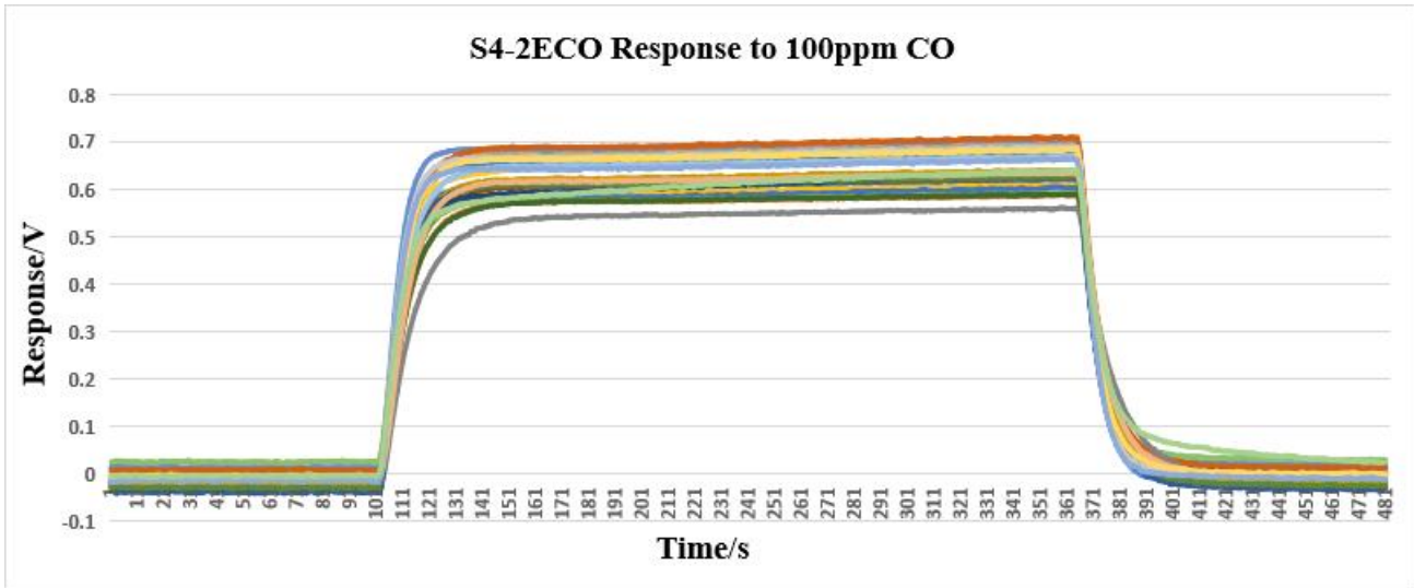
传感器响应恢复曲线 (放大电阻 150K)
