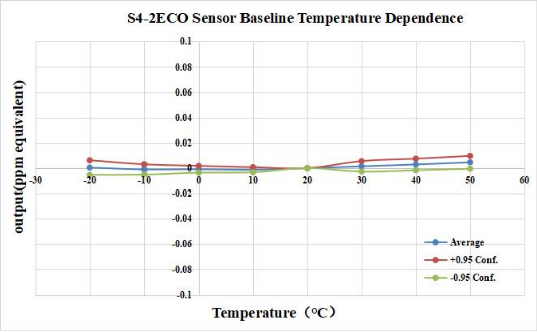
传感器基线温度特性曲线 (放大电阻 150K)
