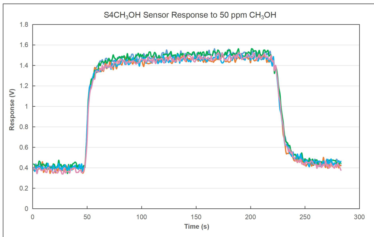
S4CH 3 OH 甲醇传感器响应恢复曲线
